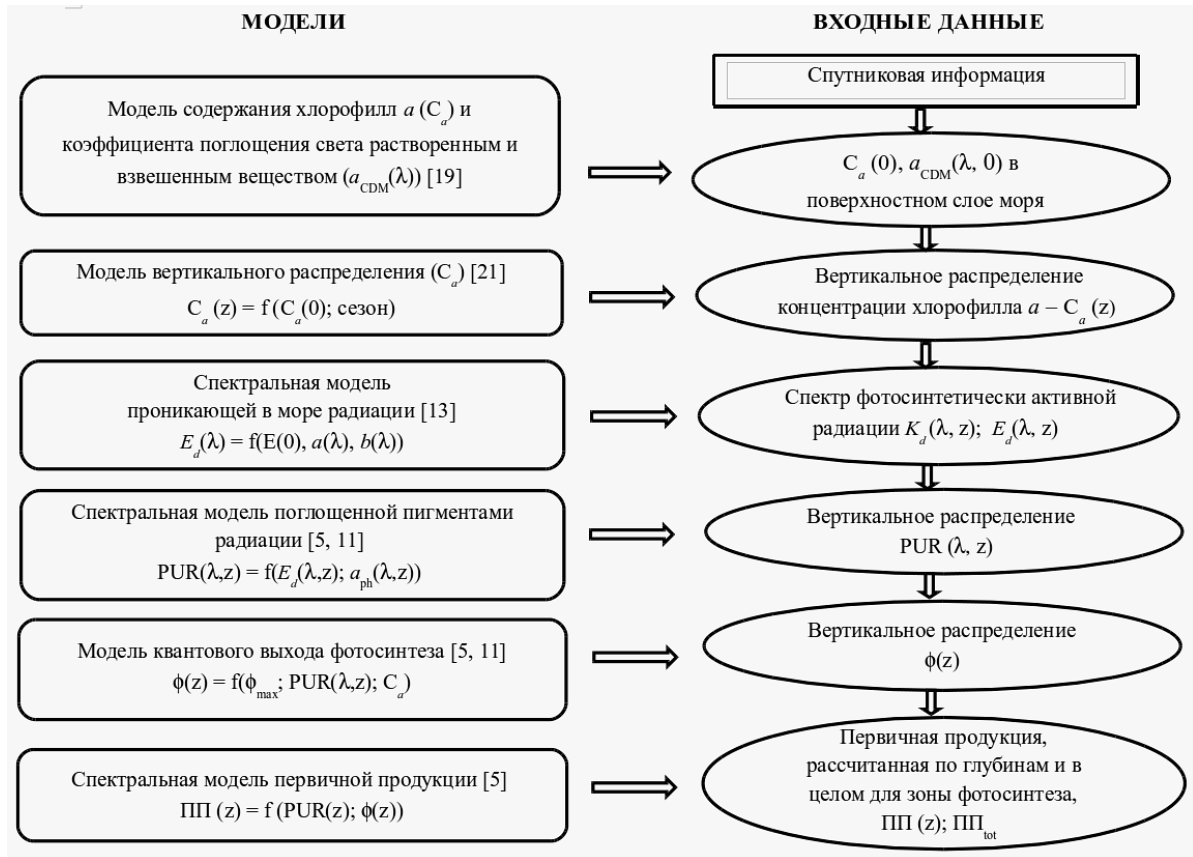
Рис. 1. Блок-схема оценки первичной продукции Чёрного моря по спутниковым данным на основе спектрального подхода, где z — глубина; a(\lambda) и \beta(\lambda) — коэффициенты поглощения и рассеяния света на длине волны — \lambda ; K_d(\lambda, z) — показатель диффузного ослабления света
